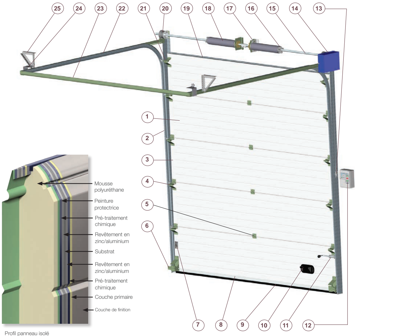
Profil panneau isolé
