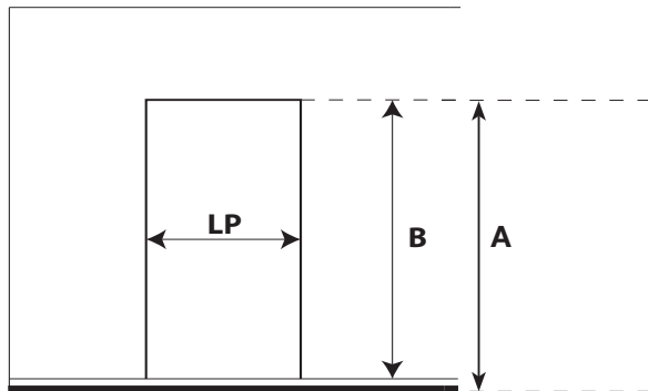
Dimension de passage du portillon
